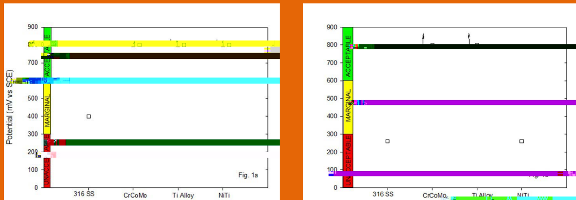
Fig.1 - Potenziali di pitting in SBF a 38°C di biomateriali: a) Test potenziodinamico, b) Test potenziostatico di scratch / Pitting potential in SBF at 38°C of biomaterials: a) potentiodynamic test, b) potentiostatic scratch test.
